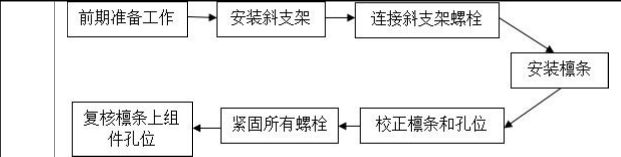
图 2-2 太阳电池组件支架安装工艺
