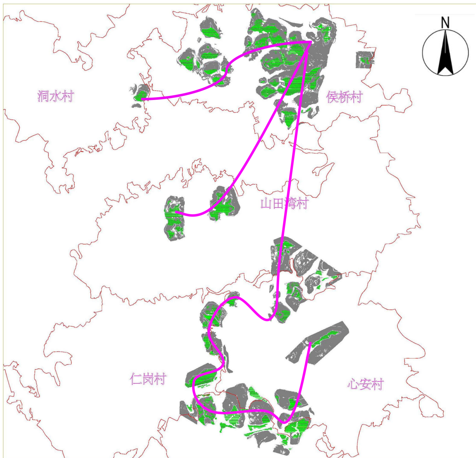
附图 4 项目集电线路图
